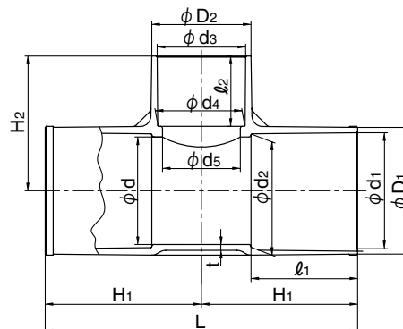
HITS HI-PVC
