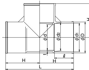
HITS HI-PVC
