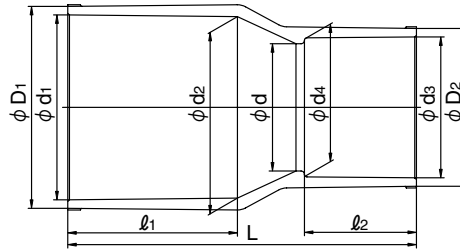
HITS HI-PVC
